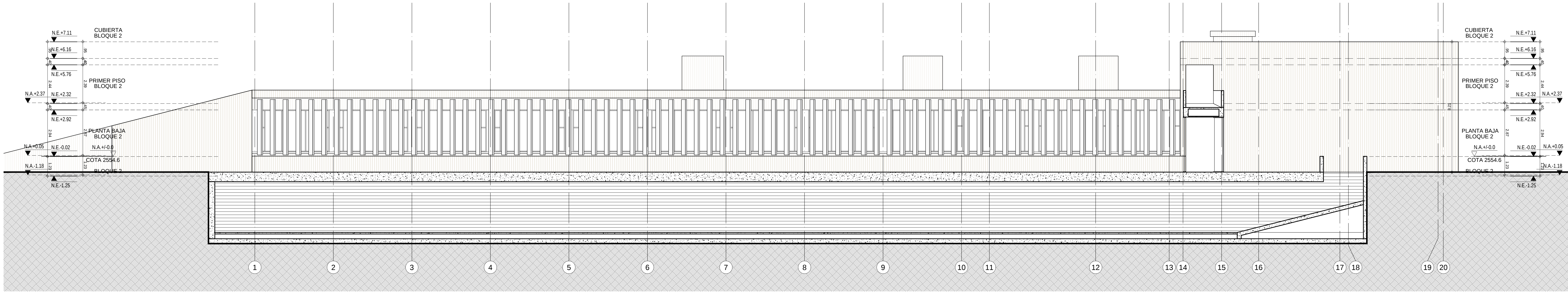
FACHADA 1 ESC. 1 : 100
